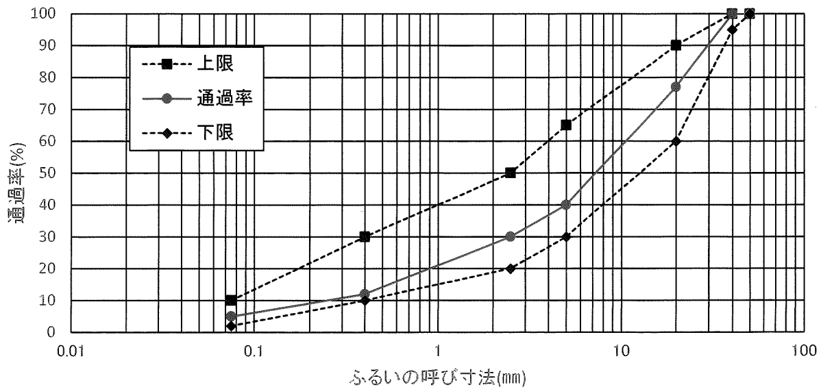
粒度曲線
