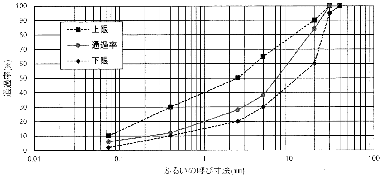
粒度曲線
