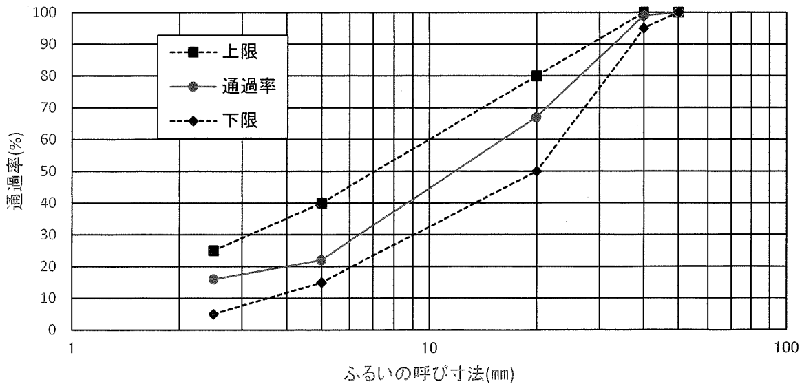
粒度曲線
