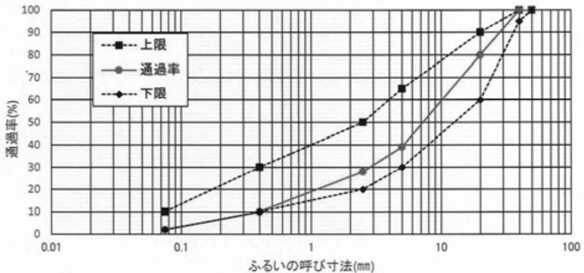
粒度曲線
