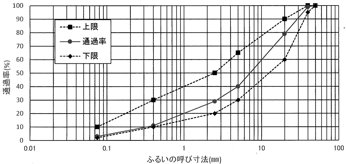
粒度曲線
