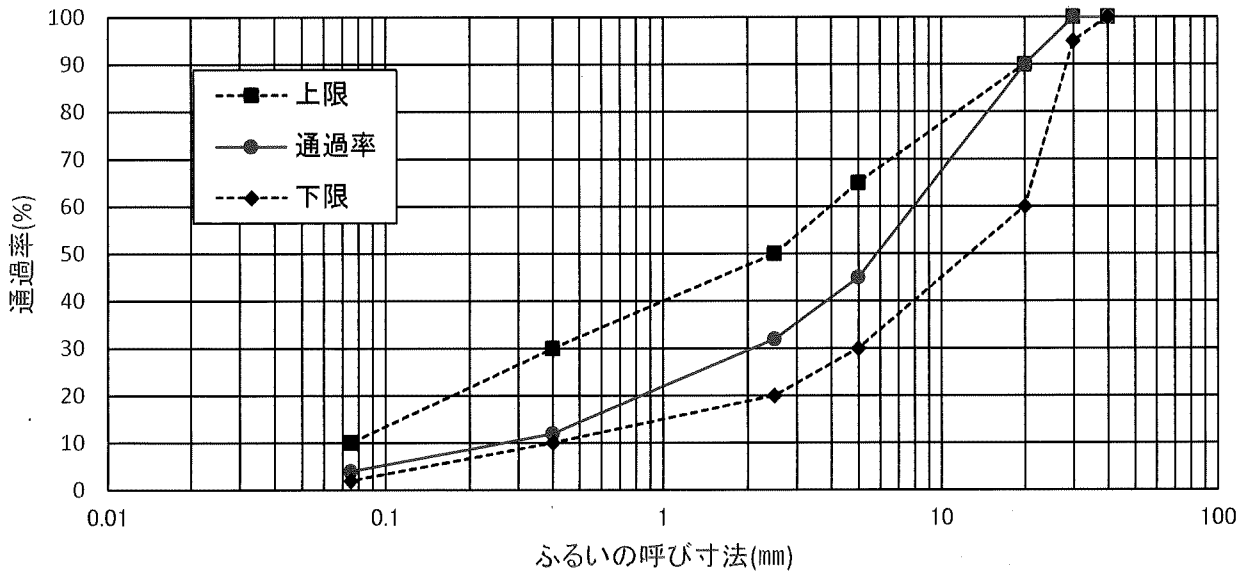
粒度曲線
